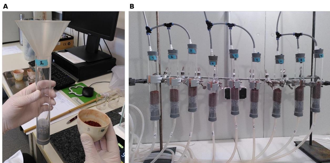
Abbildung 1: Karbonationsversuche an der BOKU an Klärschlammasche, die von BUT produziert wurde. A) Befüllung einer vorbereiteten Säule mit befeuchteter Asche; B) Durchführung der Durchfluss-Karbonatisierungsversuche.
